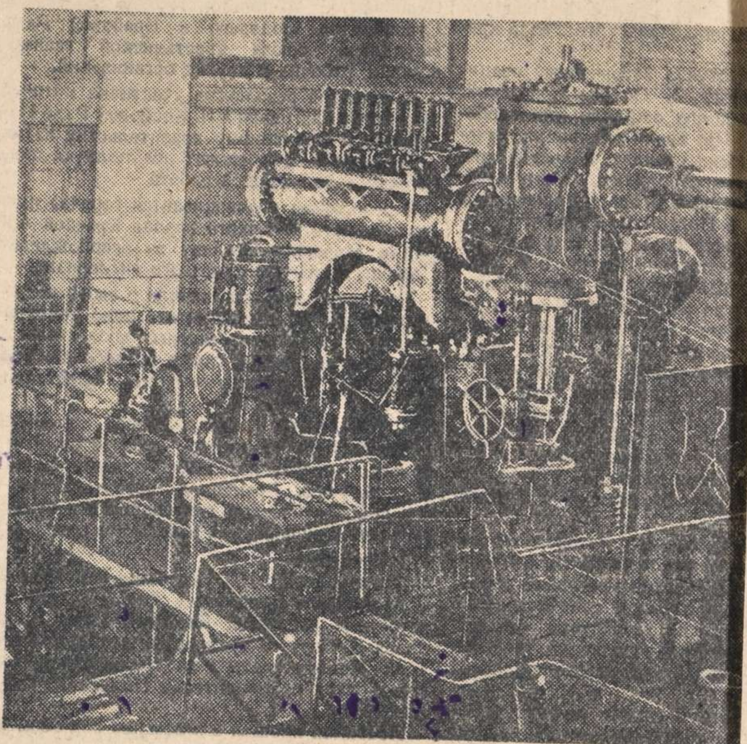
Коллектив Харьковского турбогенераторного завода им. Кирова успешно выполняет заказы для восстановления электростанций в Донбассе. На снимке — турбина мощностью в 50.000 киловатт для Зуевской ГРЭС.
