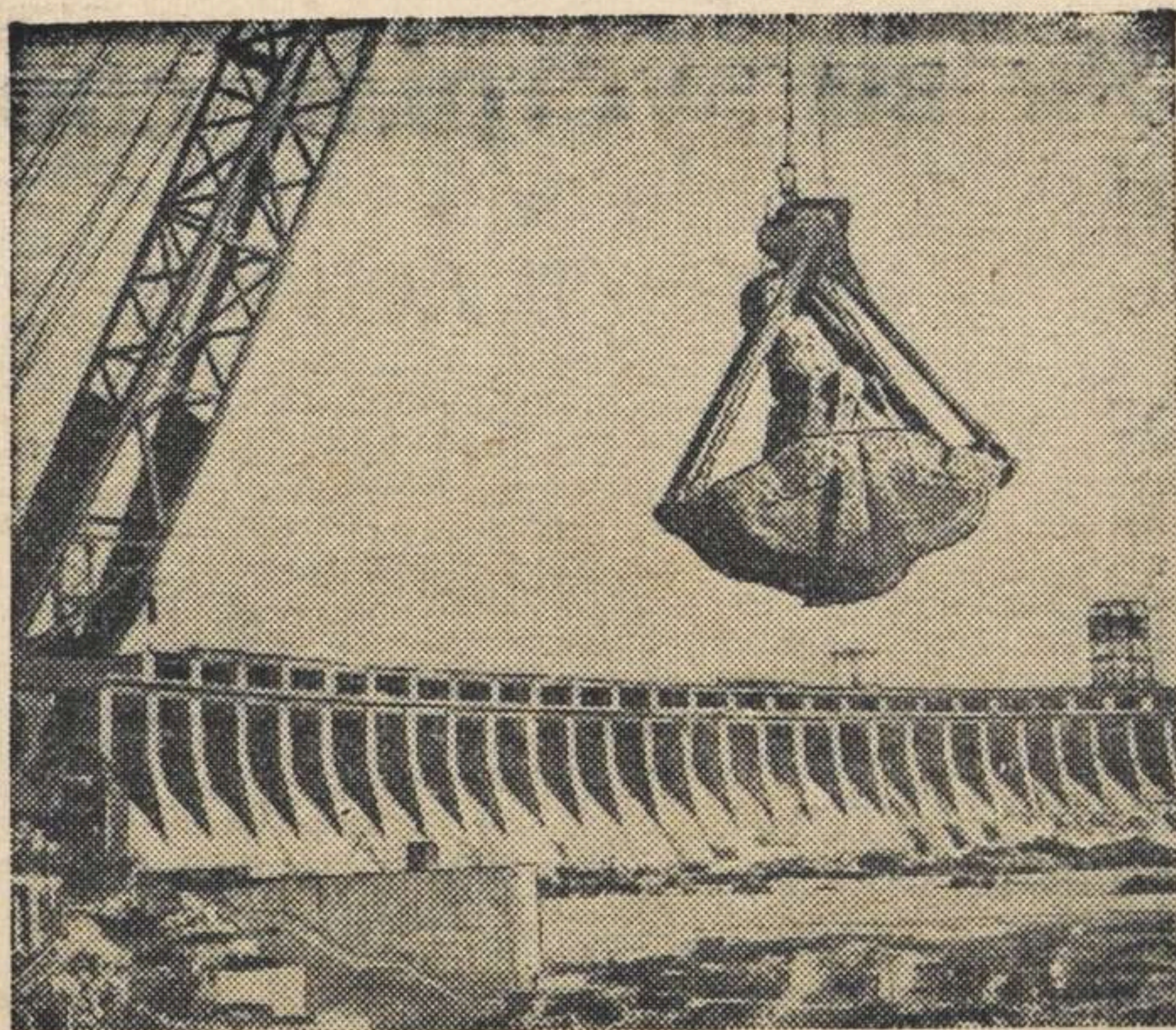
Дніпробуд. Загальний вигляд дніпровської греблі.
