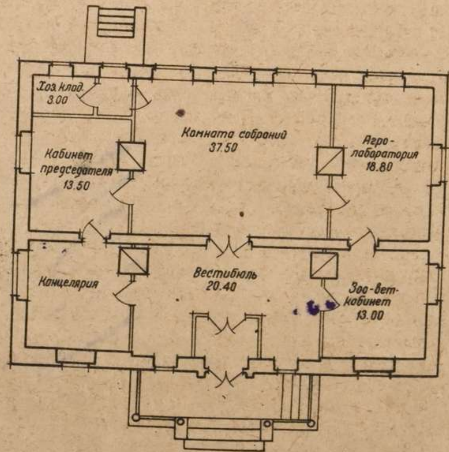
План здания конторы по проекту архитектора А. Крылова.
