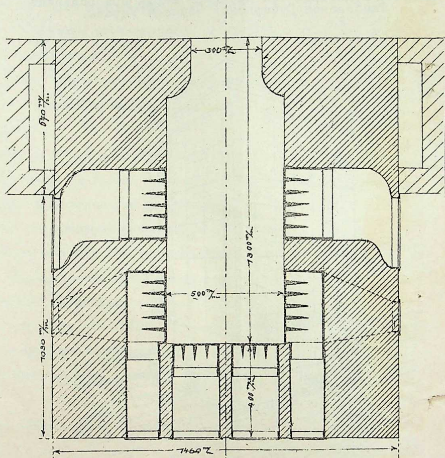
Горизонтальный разрез.
