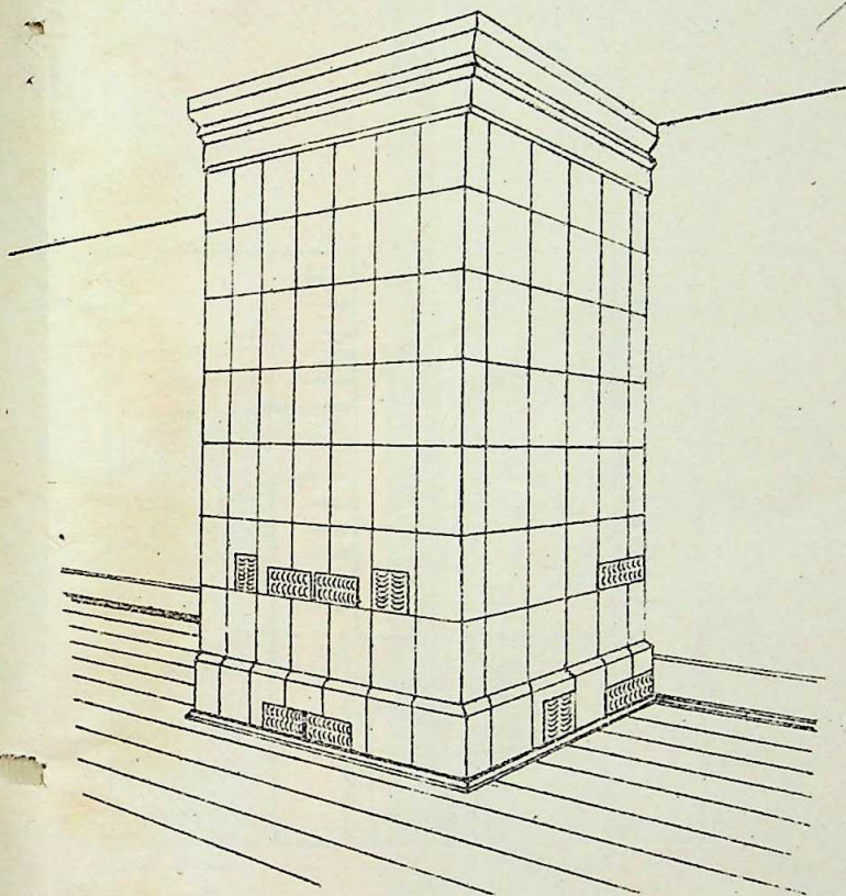
Перспективный видъ.
