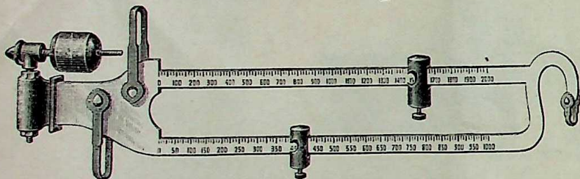
Двойное коромысло.
