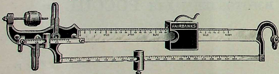
Коромысло Компаундъ.
