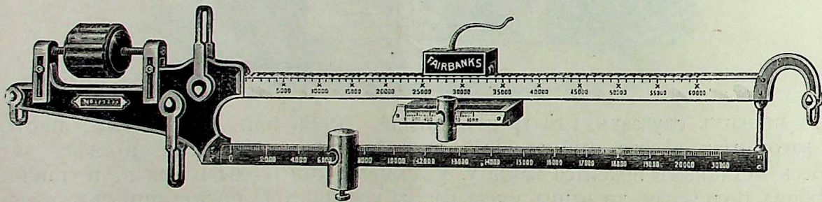
Двойное коромысло.
