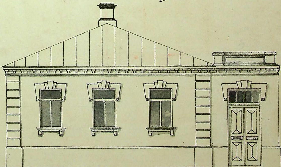
Разрѣзъ
