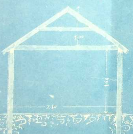
План сапожной мастерской № II
