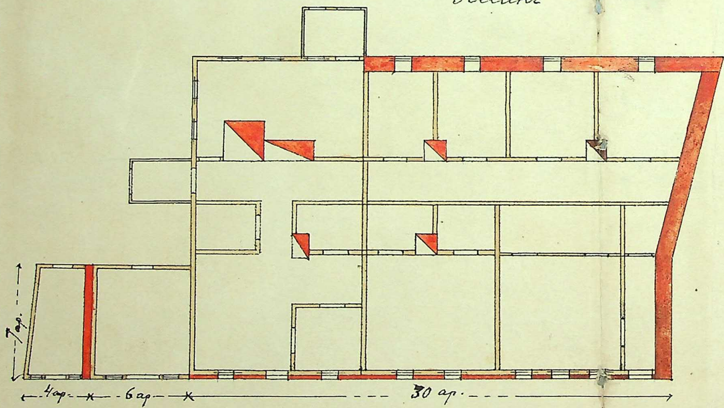
План
