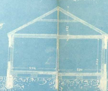
Разрез здания № II по В-В
