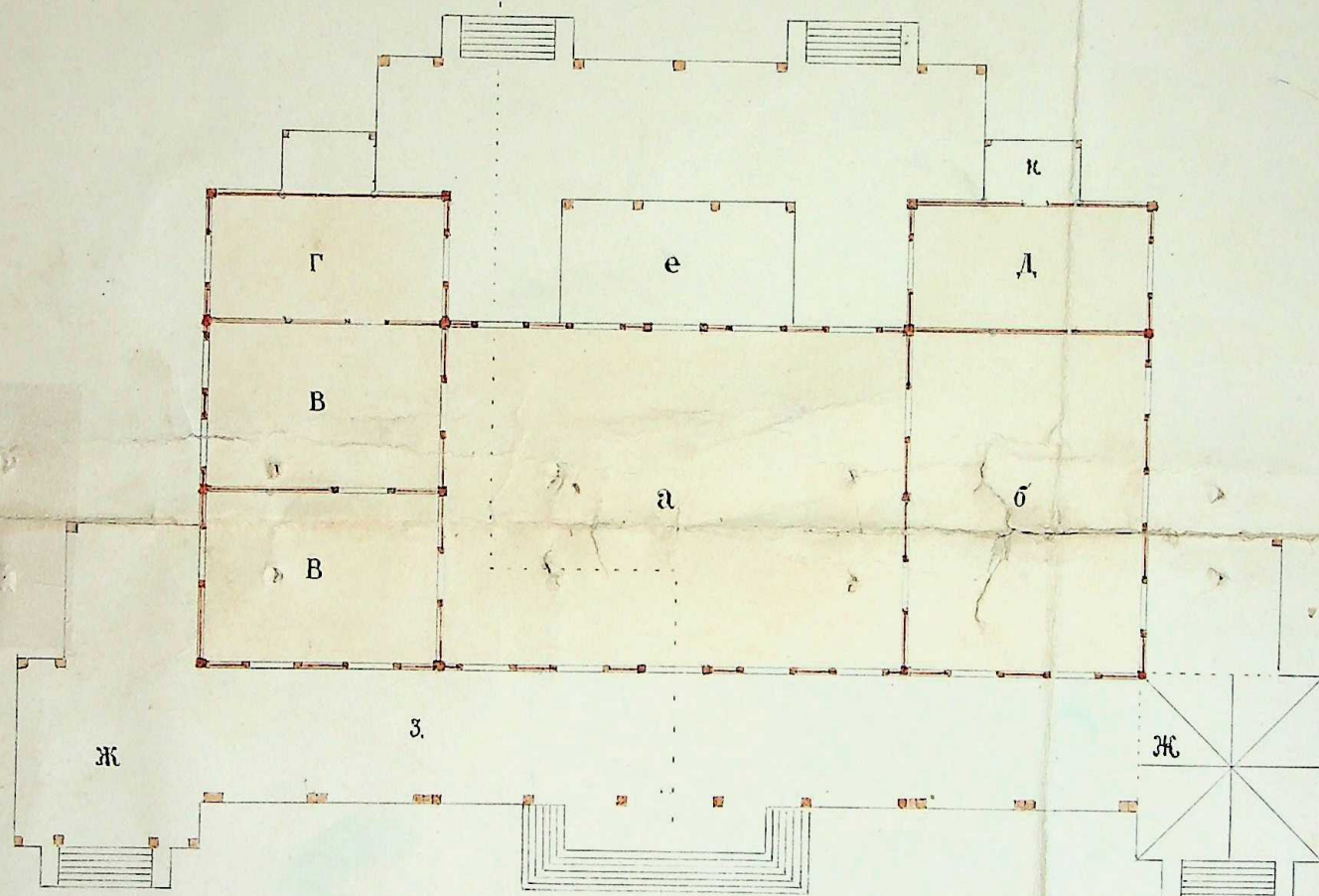
Планъ.
