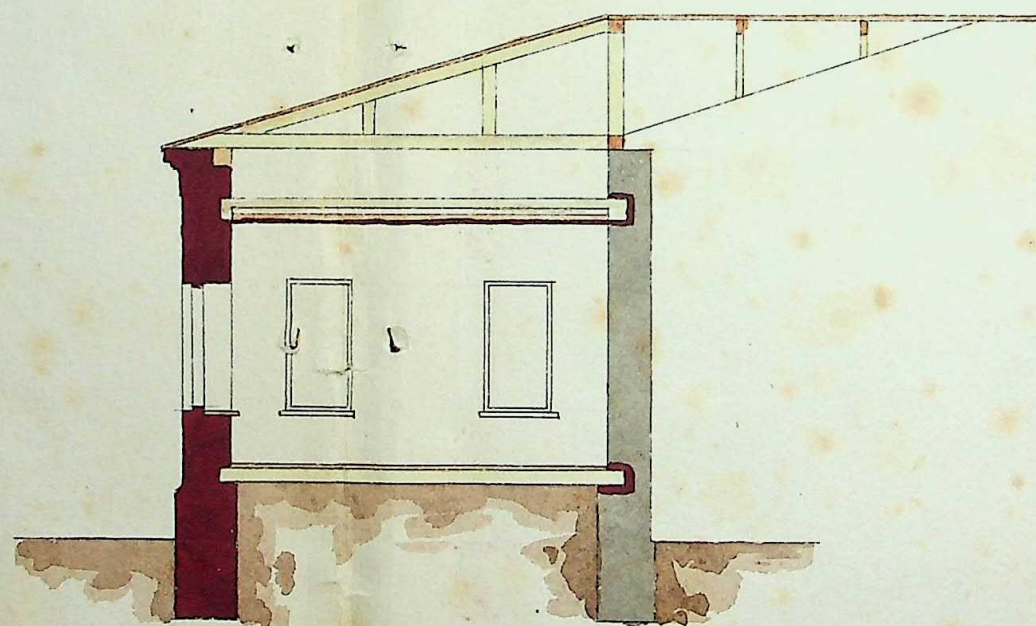
Разрѣзъ
