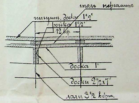
Деталь пола.
