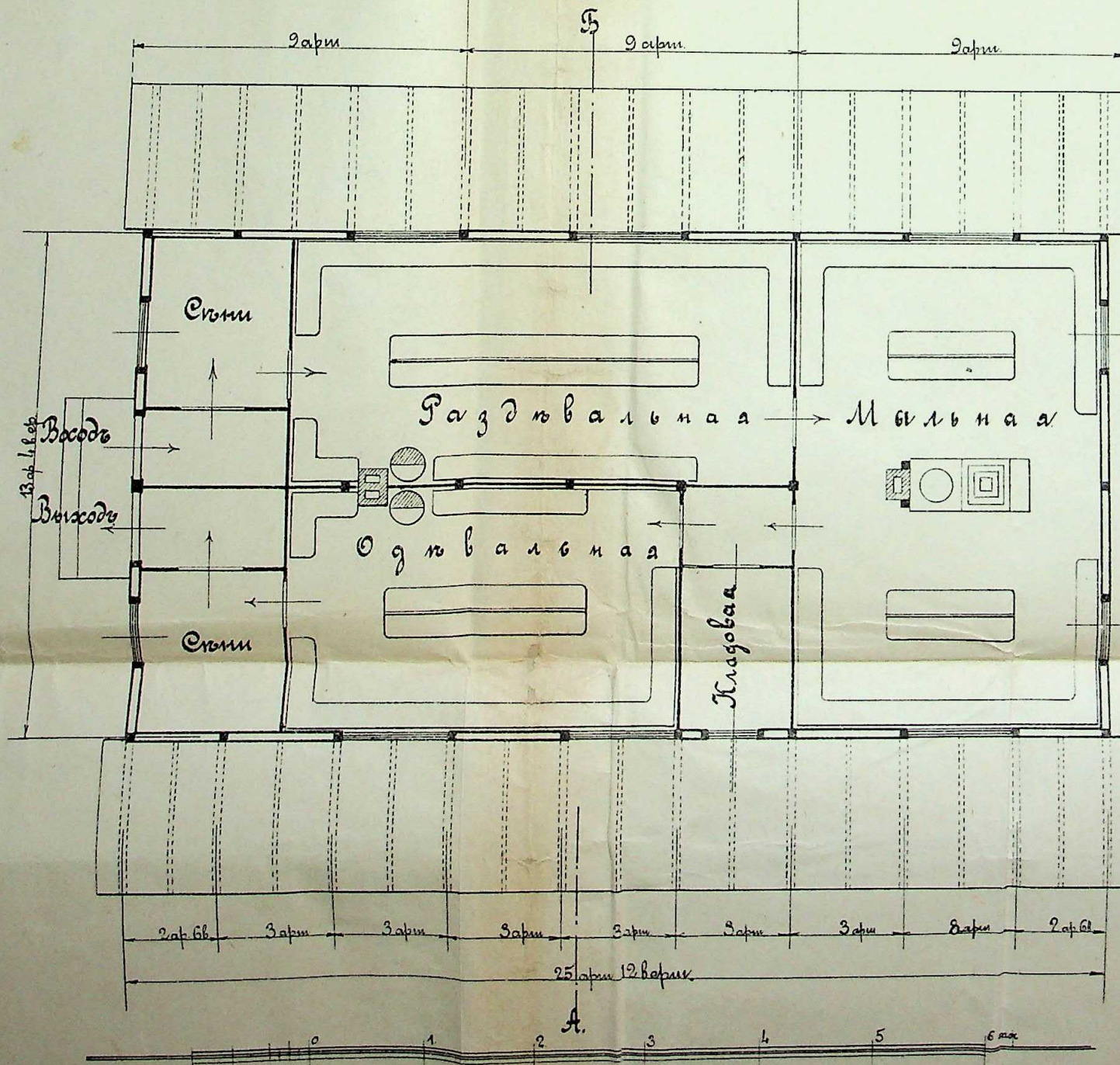
План.
