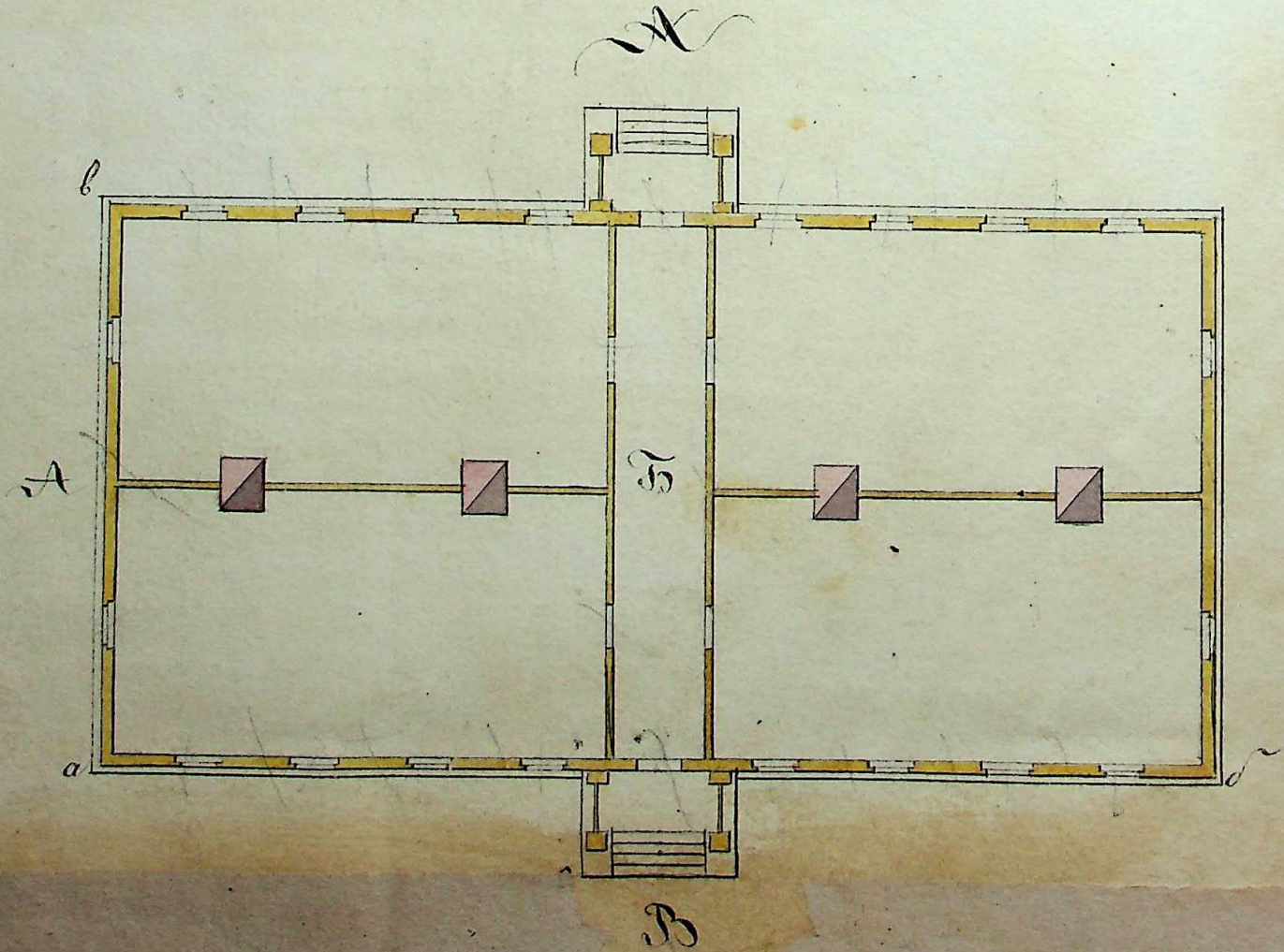
Планъ корпуса мин.
