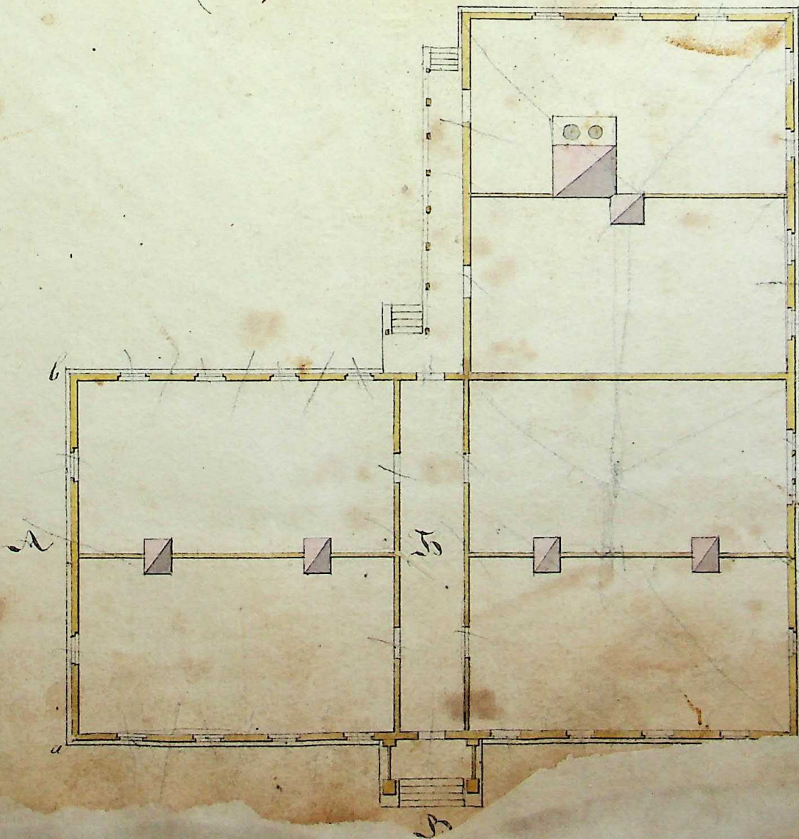
Планъ корпуса лит. Б.
