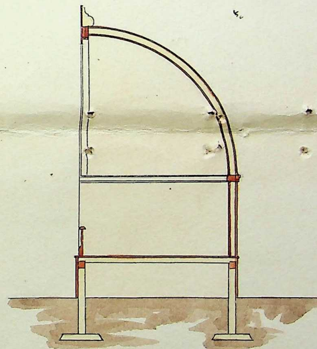
Разрѣзъ
