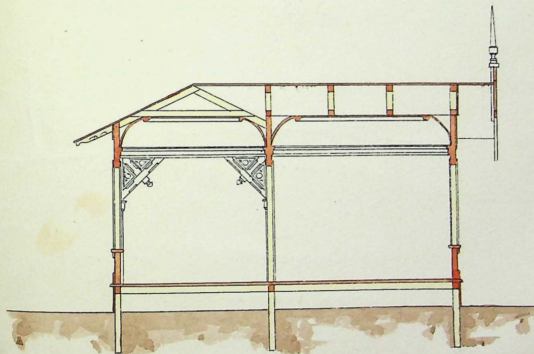
Разрѣзъ А В
